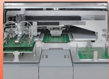
大判ワークの自動供給排出 Auto-Loading/Unloading Unit
